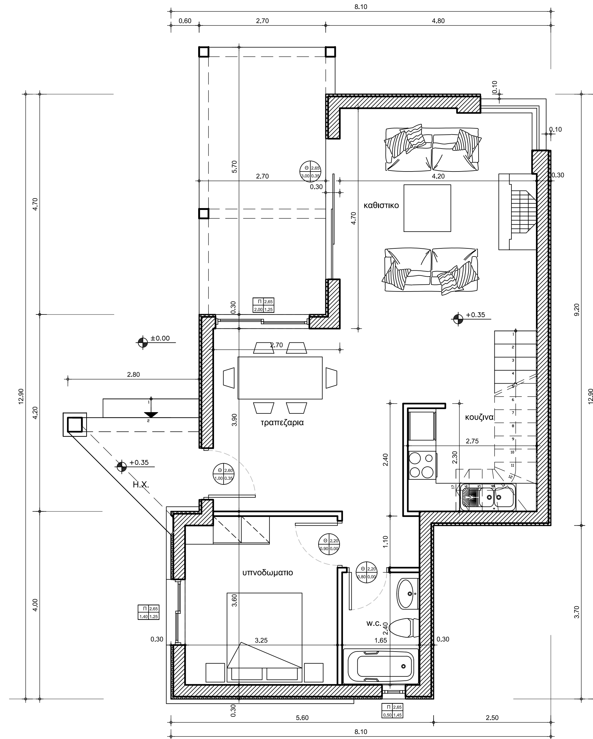
κατοψη ισογειου (κτιριο 2)
