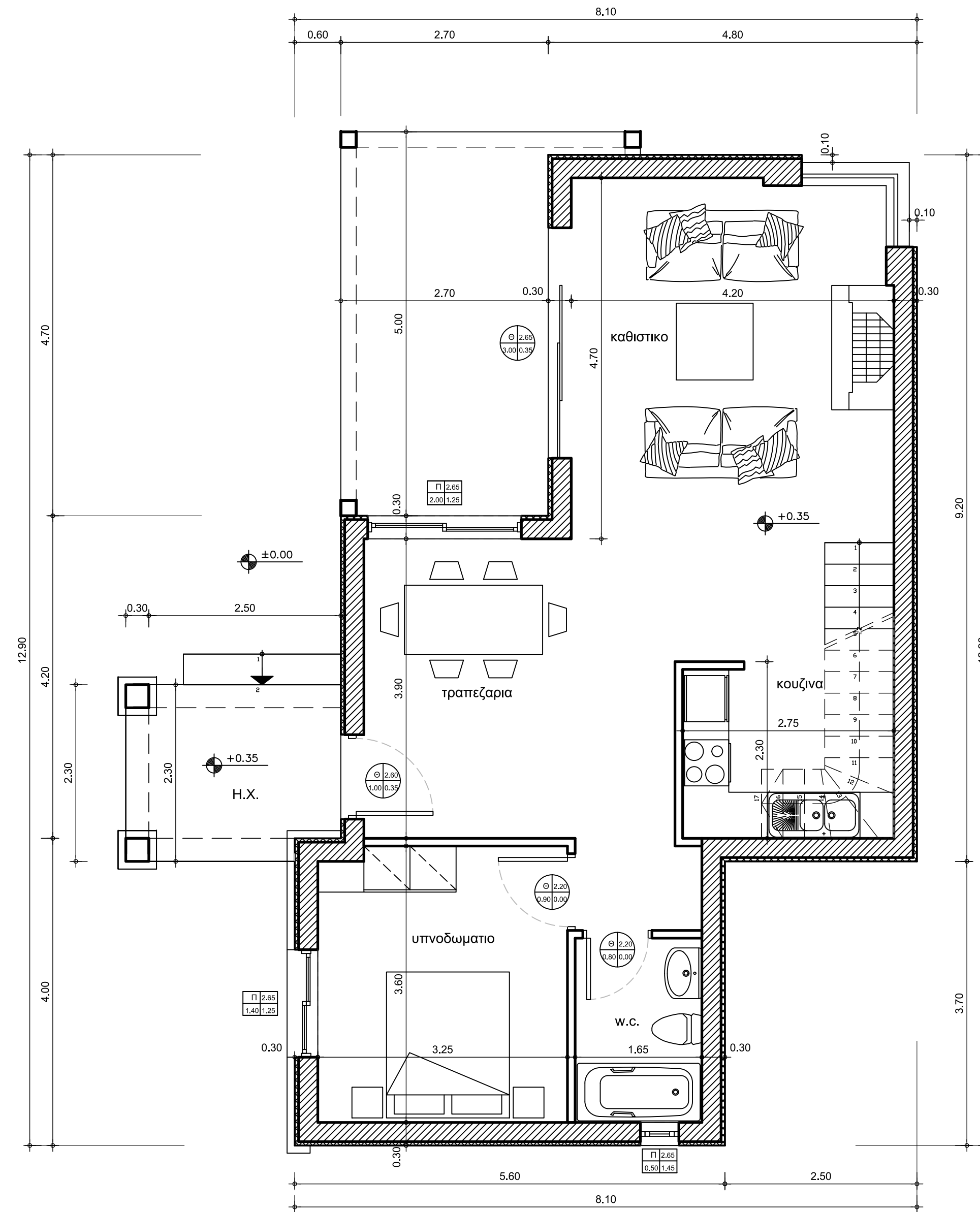
κατοψη ισουγειου (κτιριο 1)
